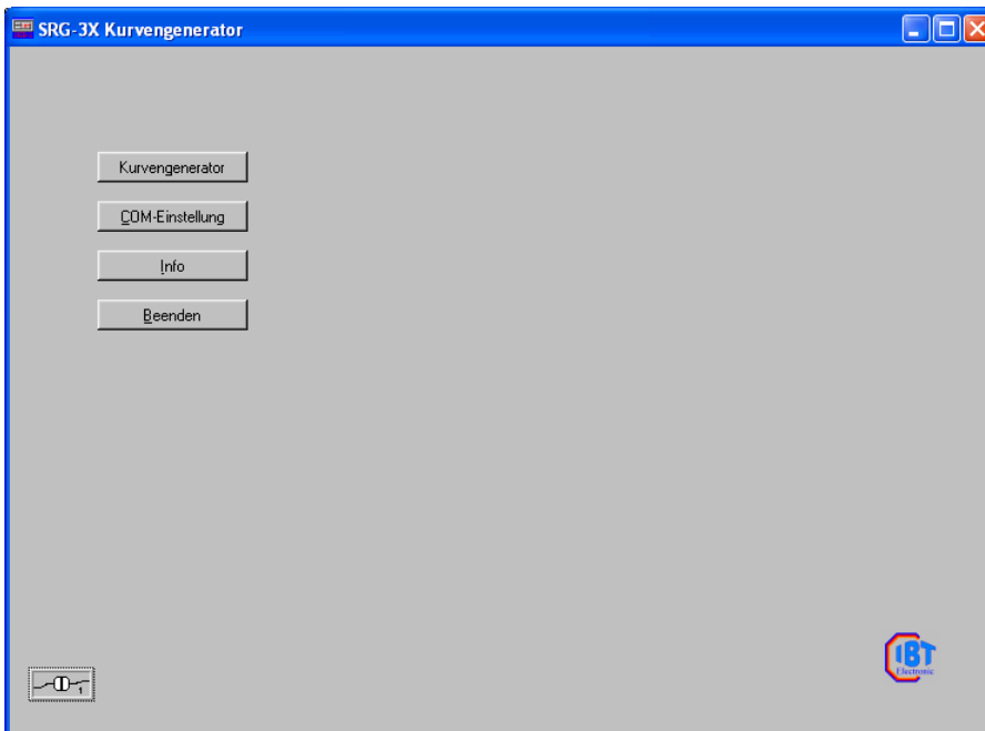
Abb. 9: Hauptfenster
