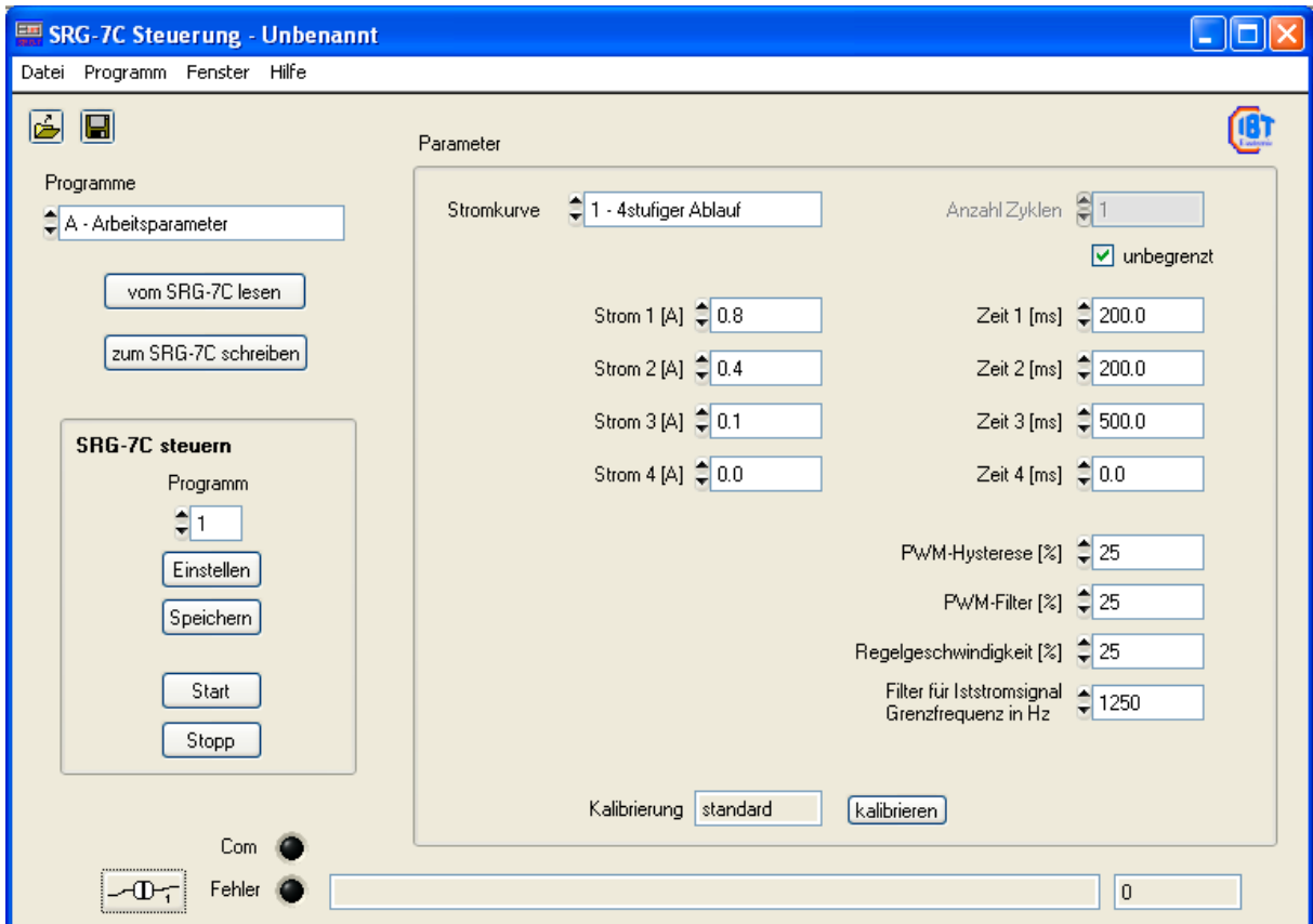
Abb. 6: Hauptfenster mit Parametereinstellung
