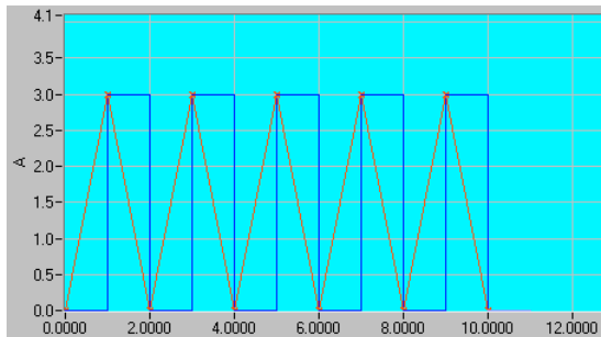
Abb. 3: 5 Rechteckimpulse
