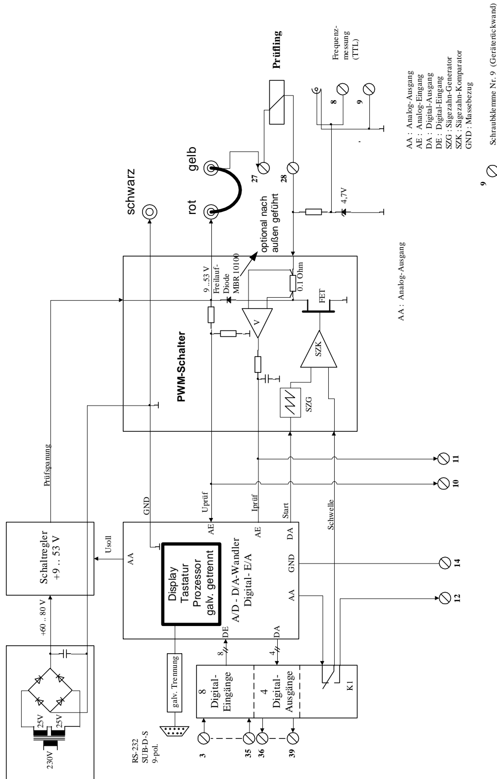
Blockschaltbild : SRG 3
